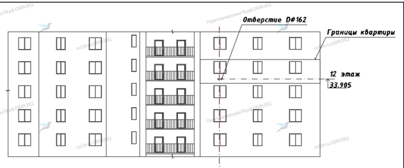
Схема крепления кондиционера к стене
