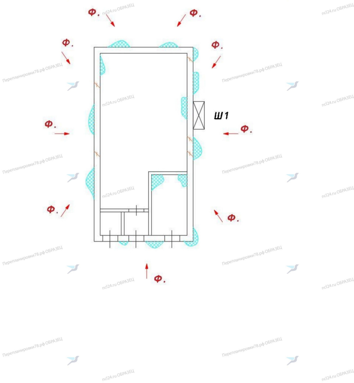
Рис. 2. План помещения. Карта дефектов и повреждений
