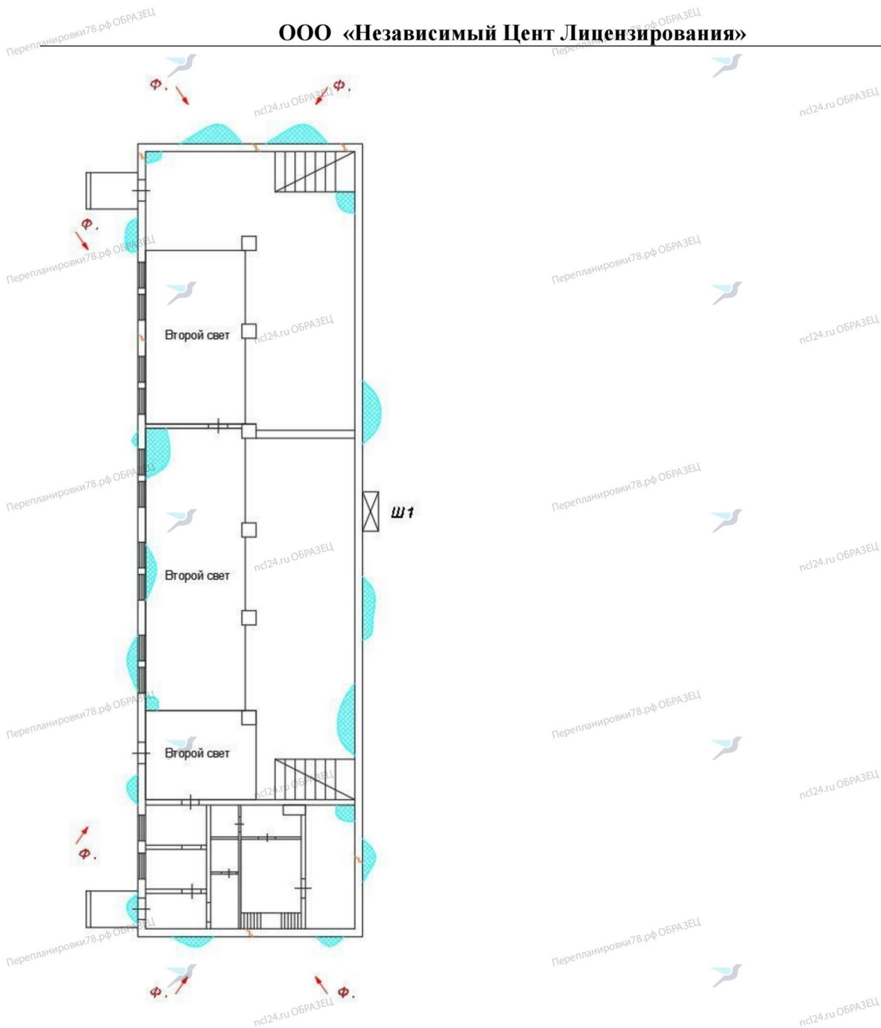
Рис. 2. План помещения. Карта дефектов и повреждений Условные обозначения:
